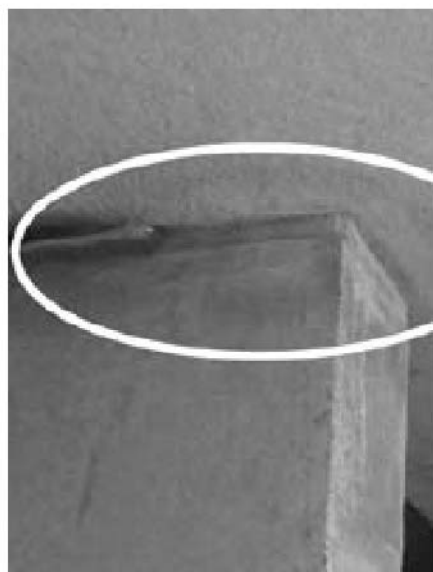
Undergjutning kortsluter flytande trapphusplan mot vägg.
