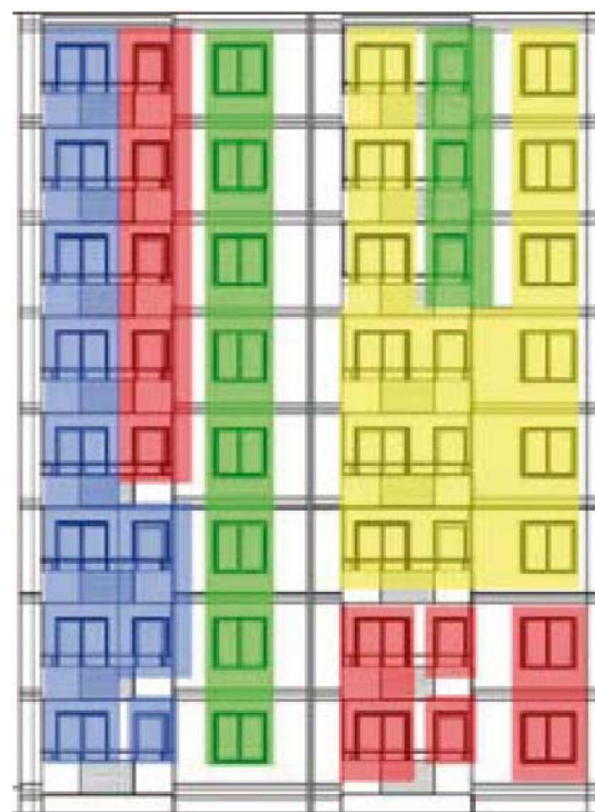
Ljudisolering R_{A,b} ( =R_w + C_b ), österfasaden: Grönt = 27; Gul = 32; Rött = 35; Blått = 38 dB.
