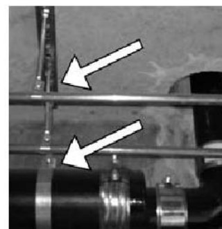
Stomljudsbyggor vid krök.
