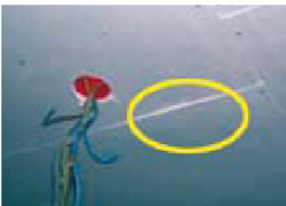
Extra skruv låser pendlad undertaksskiva mot bjälke. Källa: WSP
